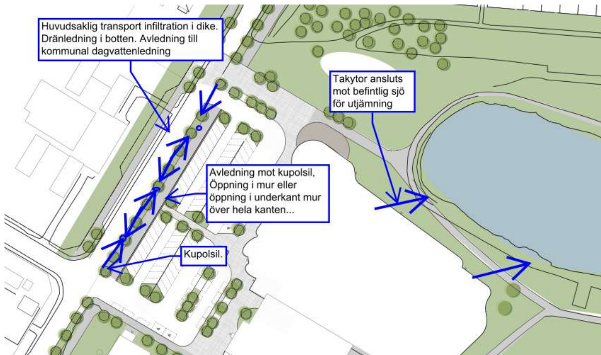
Figur 15. Exempel på fördröjande/renade åtgärder på kommande dagvattenhantering, samt tillfälligt upplag för snö. Illustrationen redovisar enbart ungefärlig placering.
