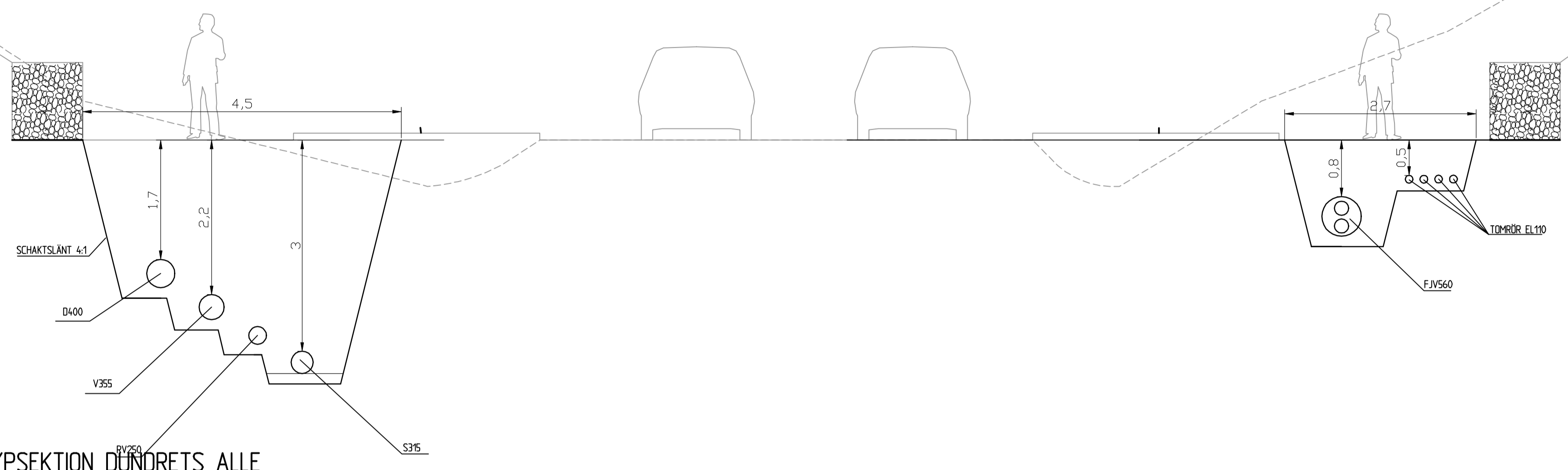
TYPSEKTION DÜNDRETS ALLE SKALA 1:50
