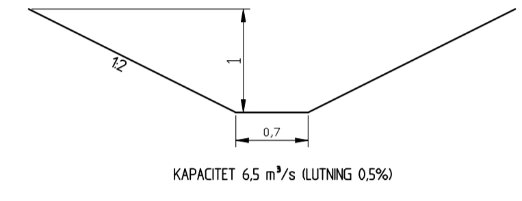
TYPSEKTION AVSKÄRANDE DIKE SKALA 1:50
