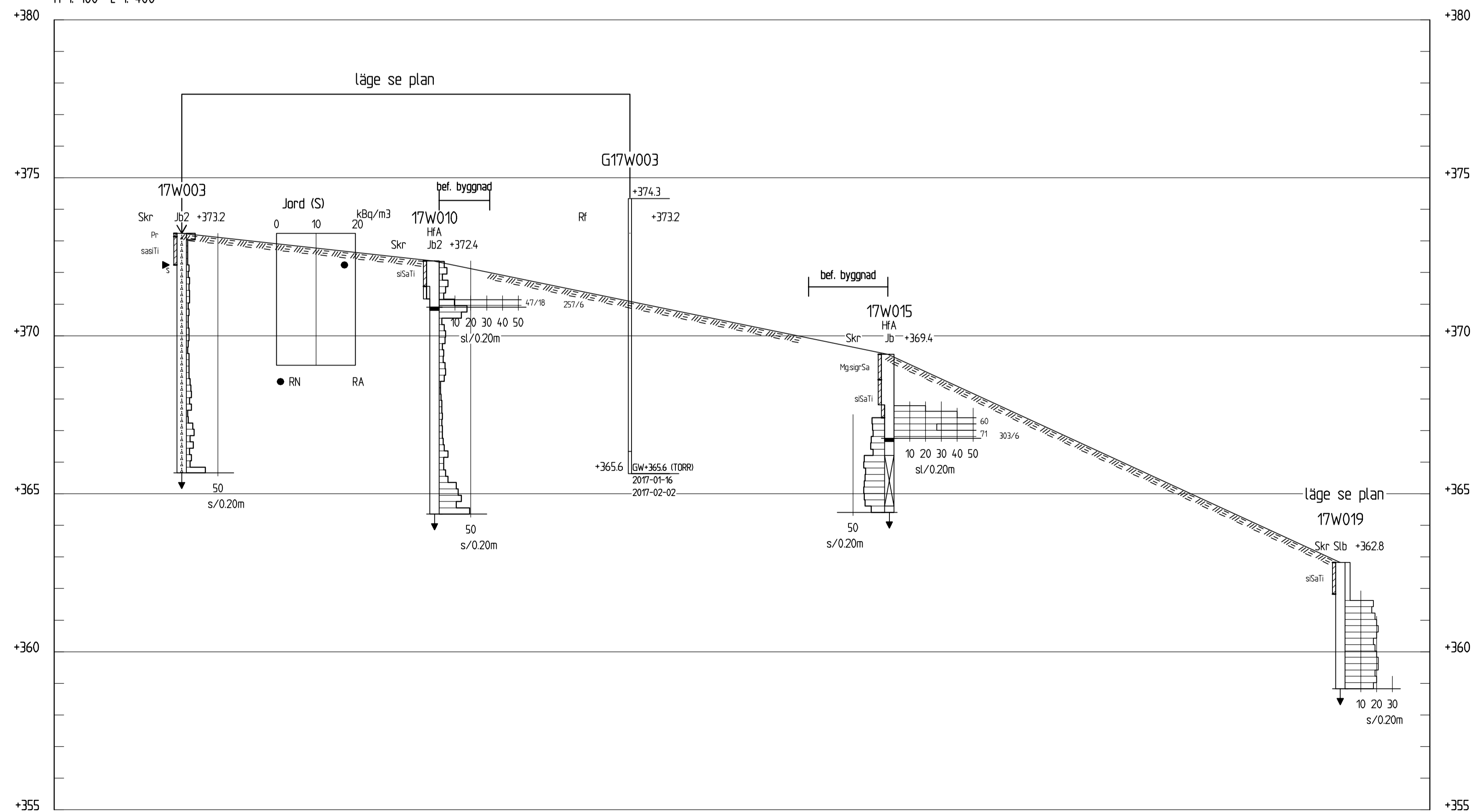
SEKTION B-B H 1:100 L 1:400
