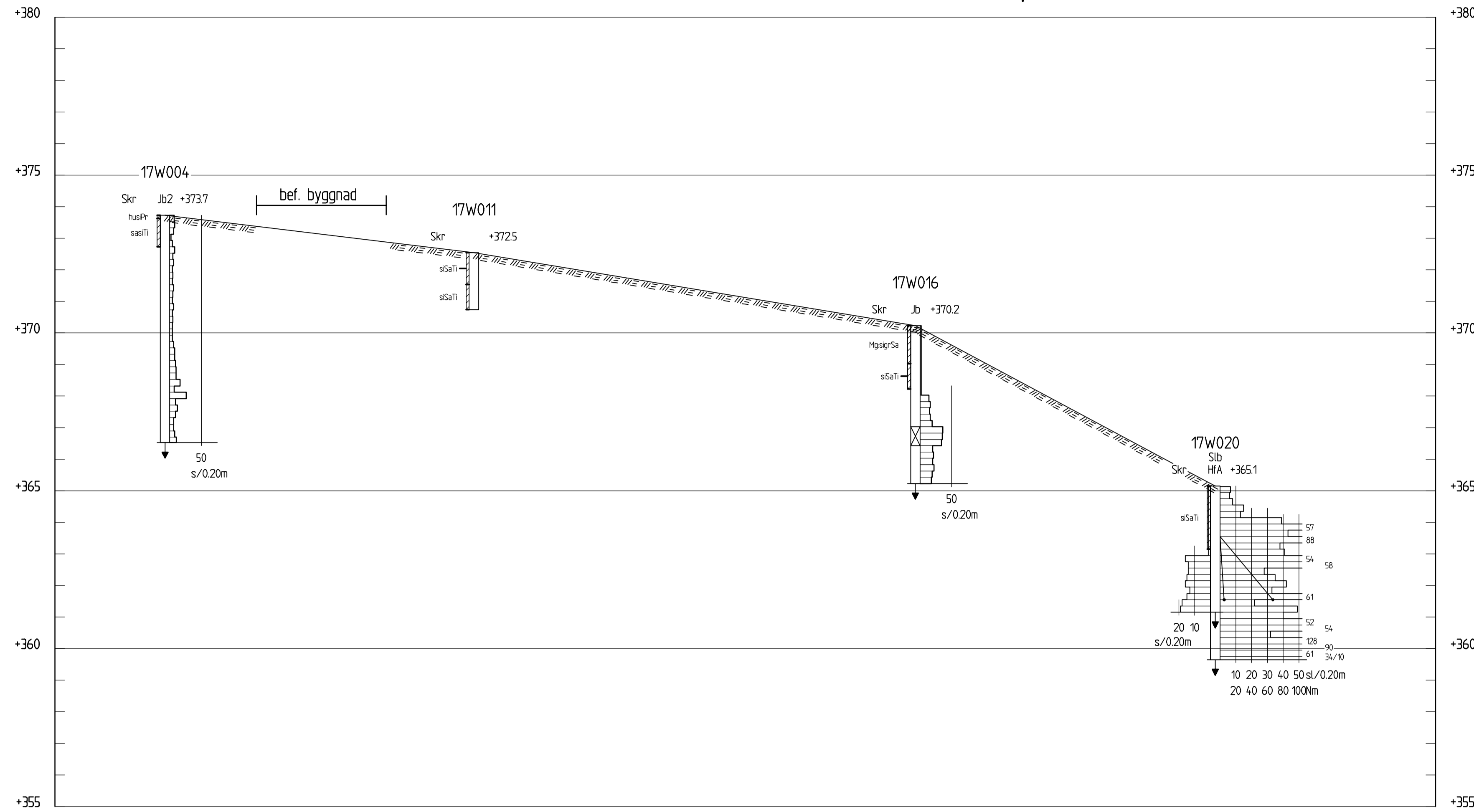
SEKTION A-A H 1:100 L 1:400
