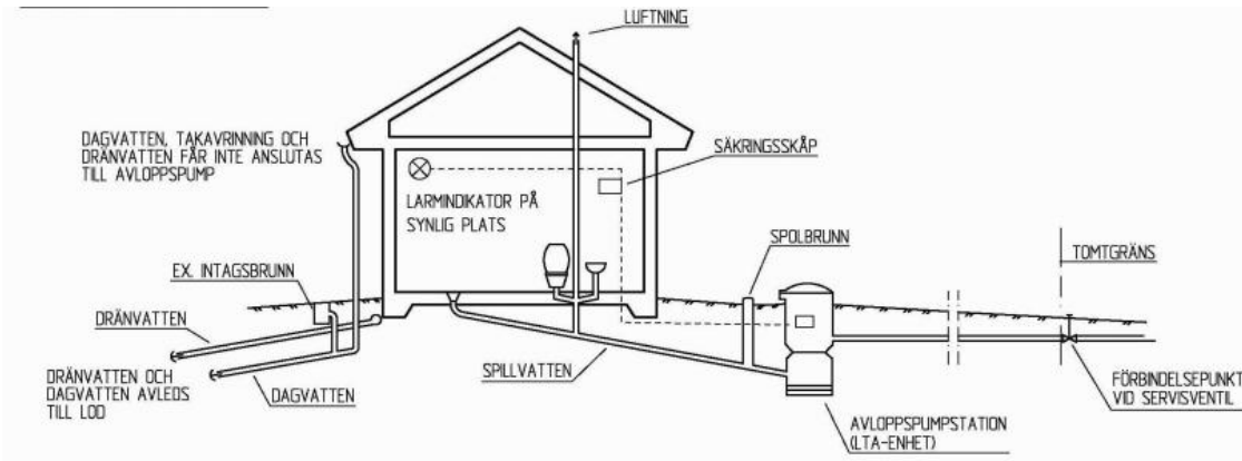
Figur 1. Principlösning LTA-system
